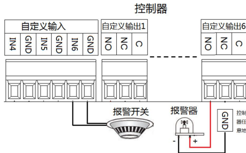
图 11：报警开关、报警灯接线示意图，有源输出接线方式
