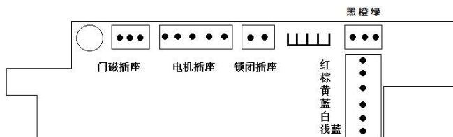
图一：DW-LDS2-K/1K
