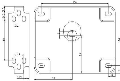
电控锁安装示意图
